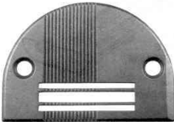
ART. 6602 - # 272-006501 leicht (light)
